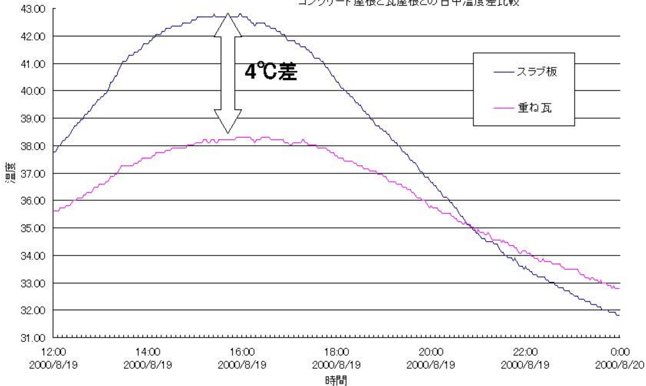
コンクリート屋根と瓦屋根との日中温度差比較
